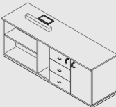
ARMÁRIO NICHOS + GAVETEIRO 3 GAVETAS + ARMÁRIO 1 PORTA LADO DIREITO L 1700 x P 500 x H 645mm APNX1705GPD
