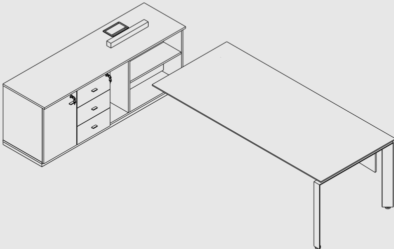
ARMÁRIO NICHOS + GAVETEIRO 3 GAVETAS LADO ESQUERDO L 1300 x P 500 x H 645mm APNX1305GE
