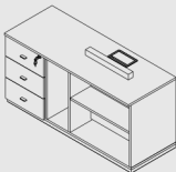
ARMÁRIO NICHOS + GAVETEIRO 3 GAVETAS LADO ESQUERDO L 1300 x P 500 x H 645mm APNX1305GE
